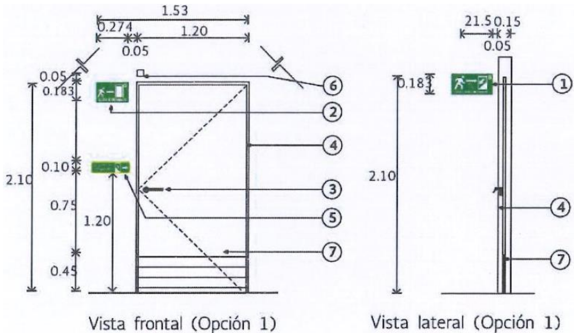
121 MEDIDAS DE SALIDAS DE EMERGENCIA (OPCIÓN 1)
